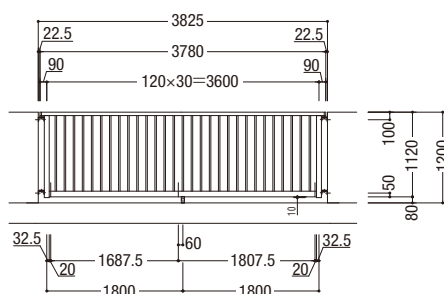
壁支持型
