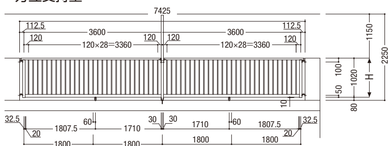
方立支持型
